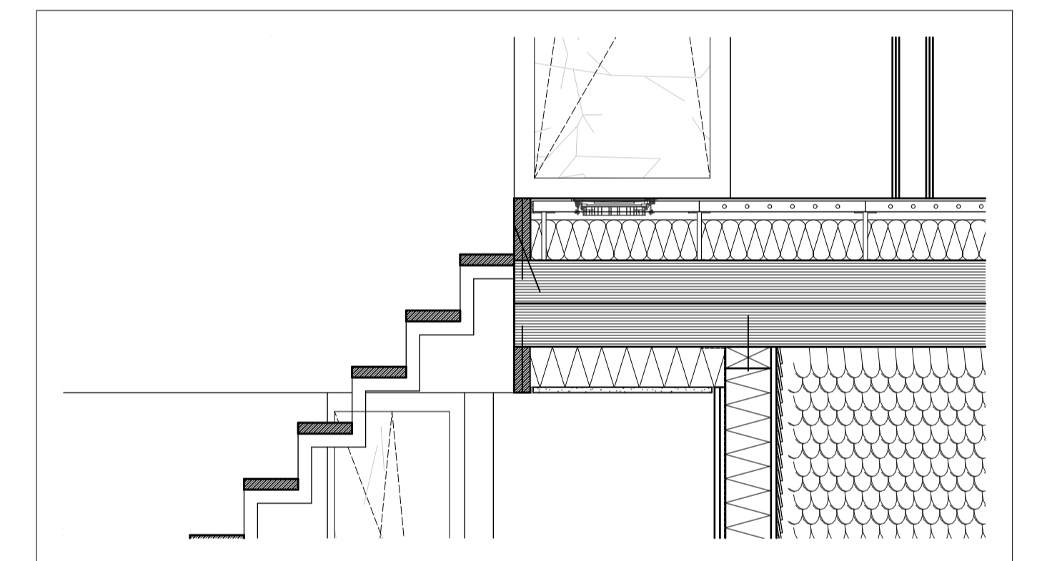
DETAIL - TREPPENAUSRITT
