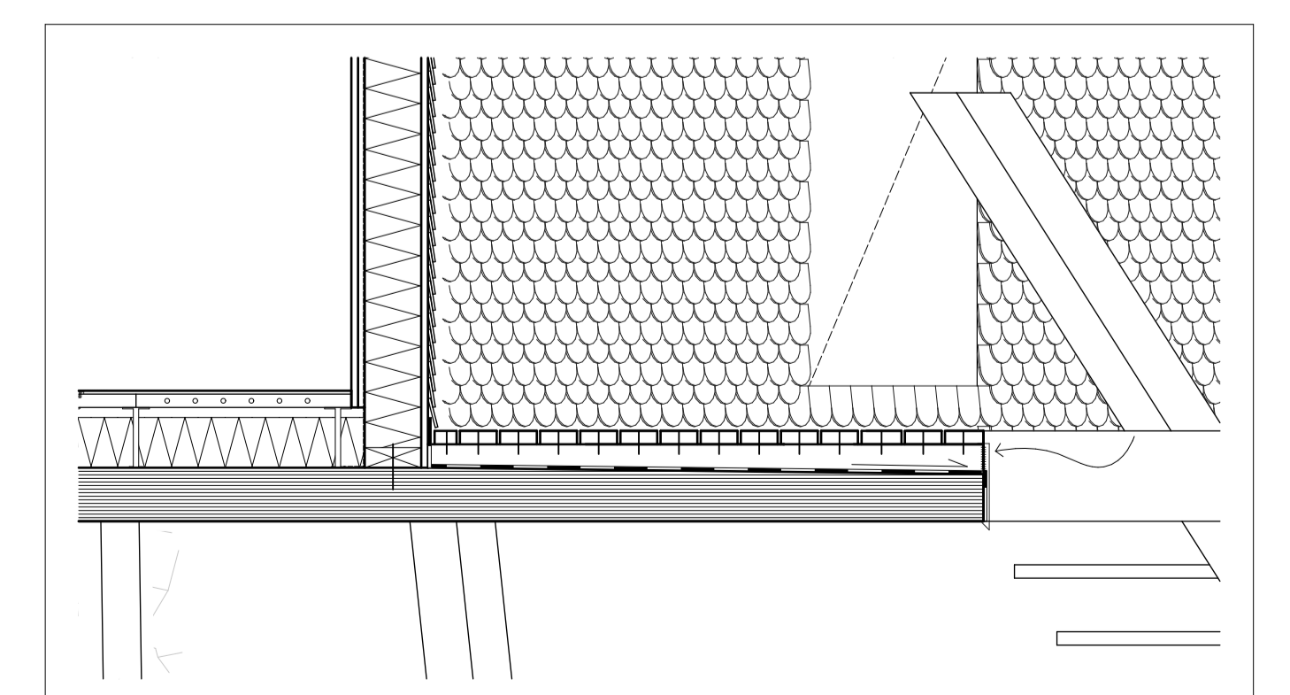
DETAIL - WANDANSCHLUSS
