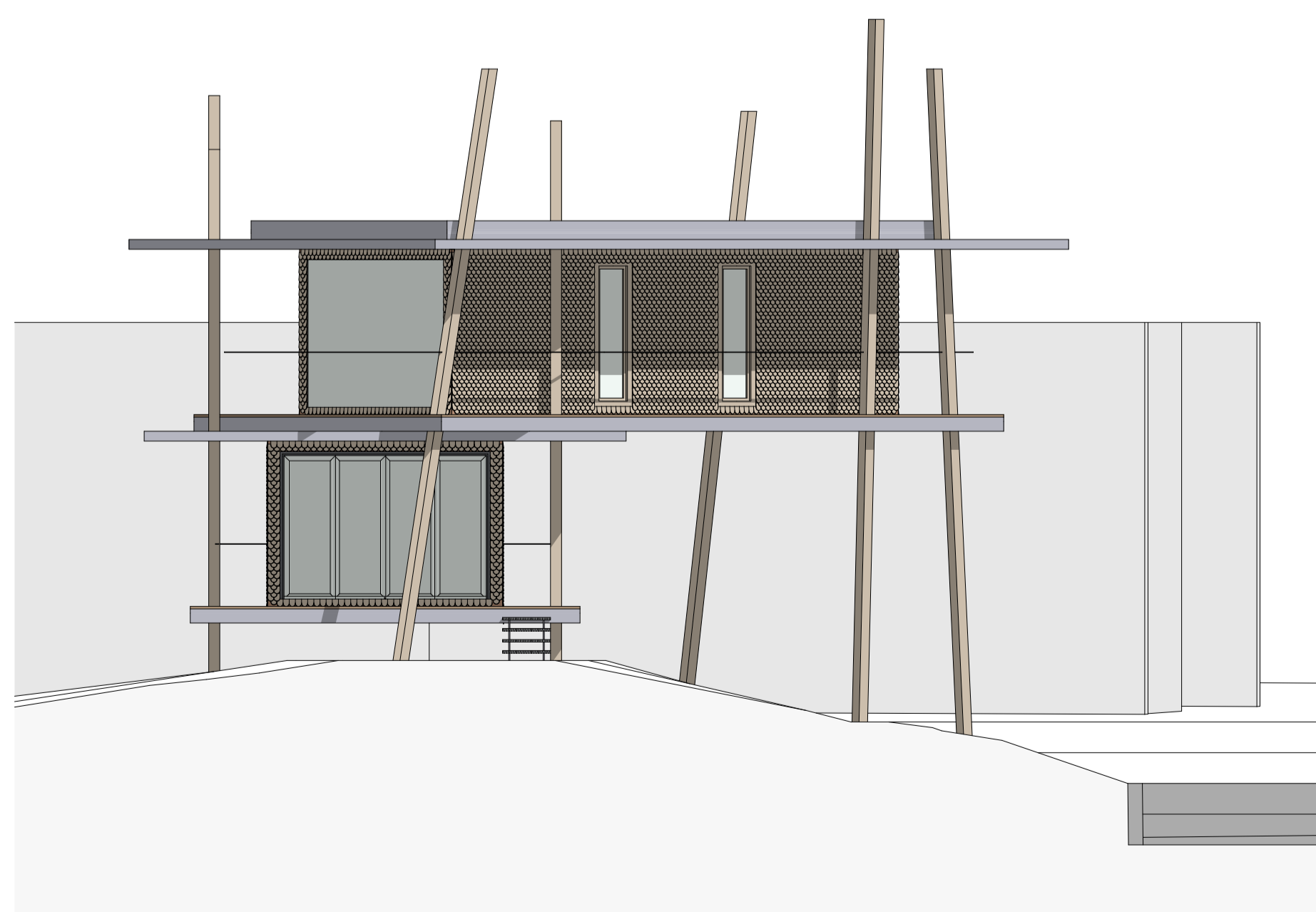
ANSICHT OST
