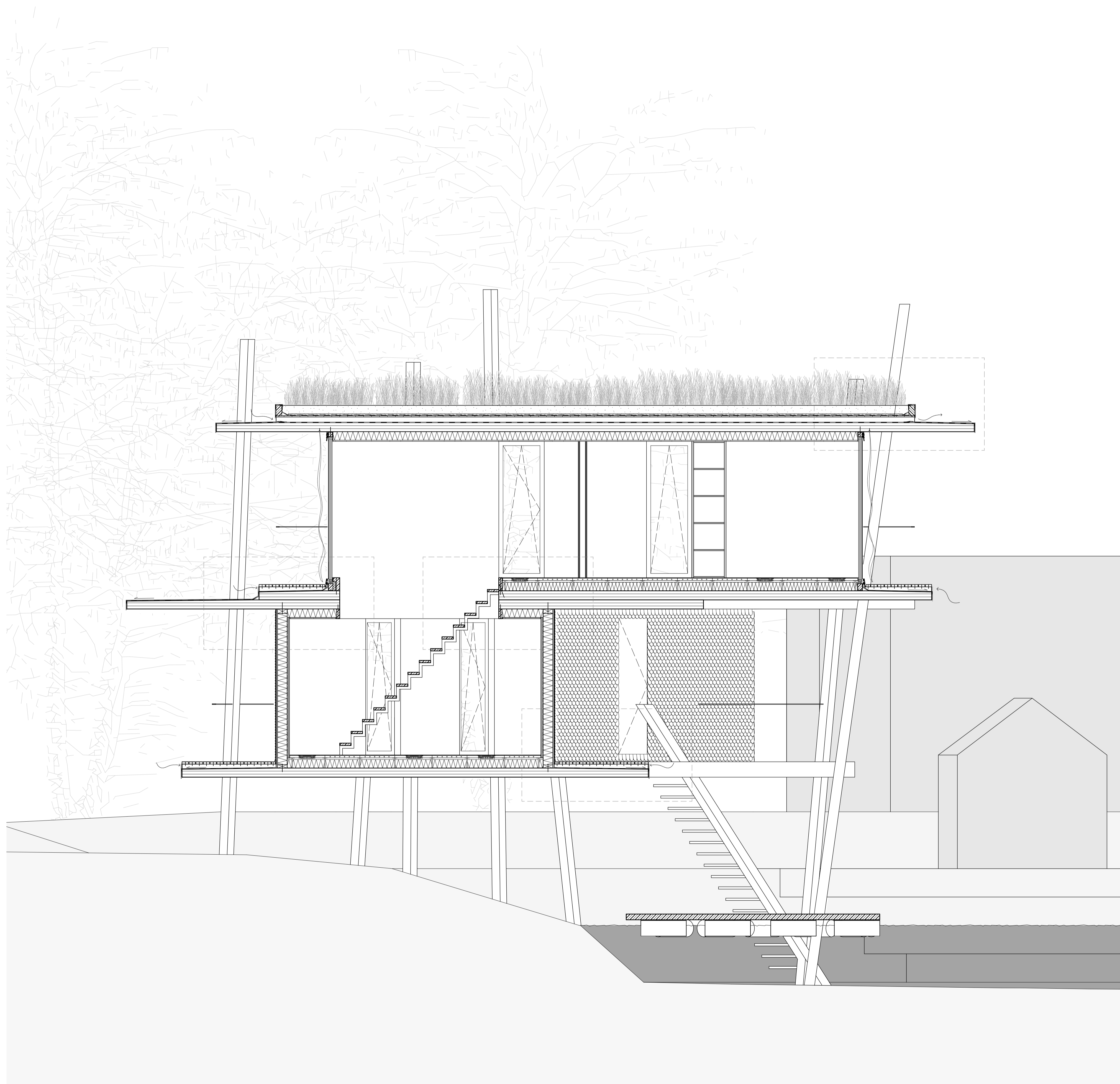
GEBÄUDEQUERSCHNITT
