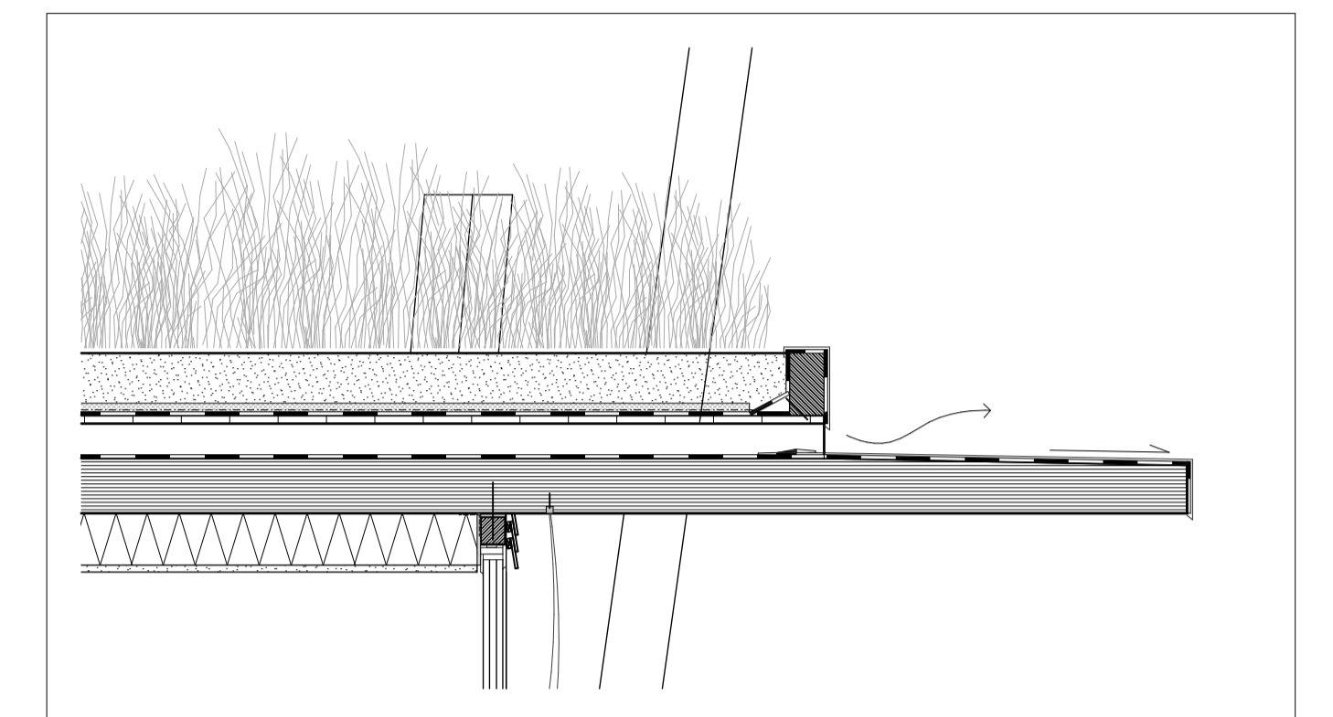
DETAIL - DACHAUFBAU
