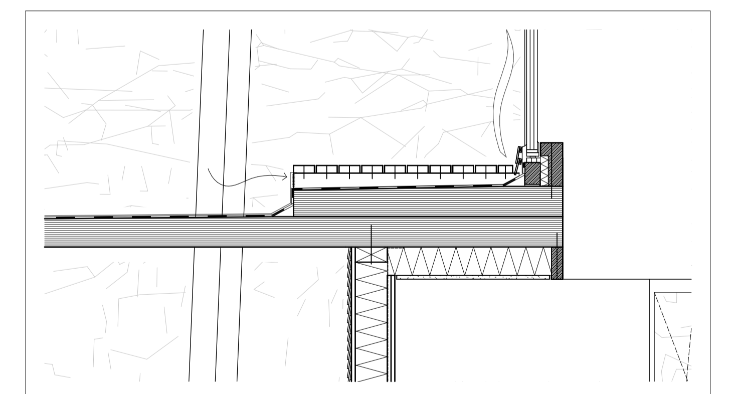
DETAIL - FENSTERANSCHLUSS
