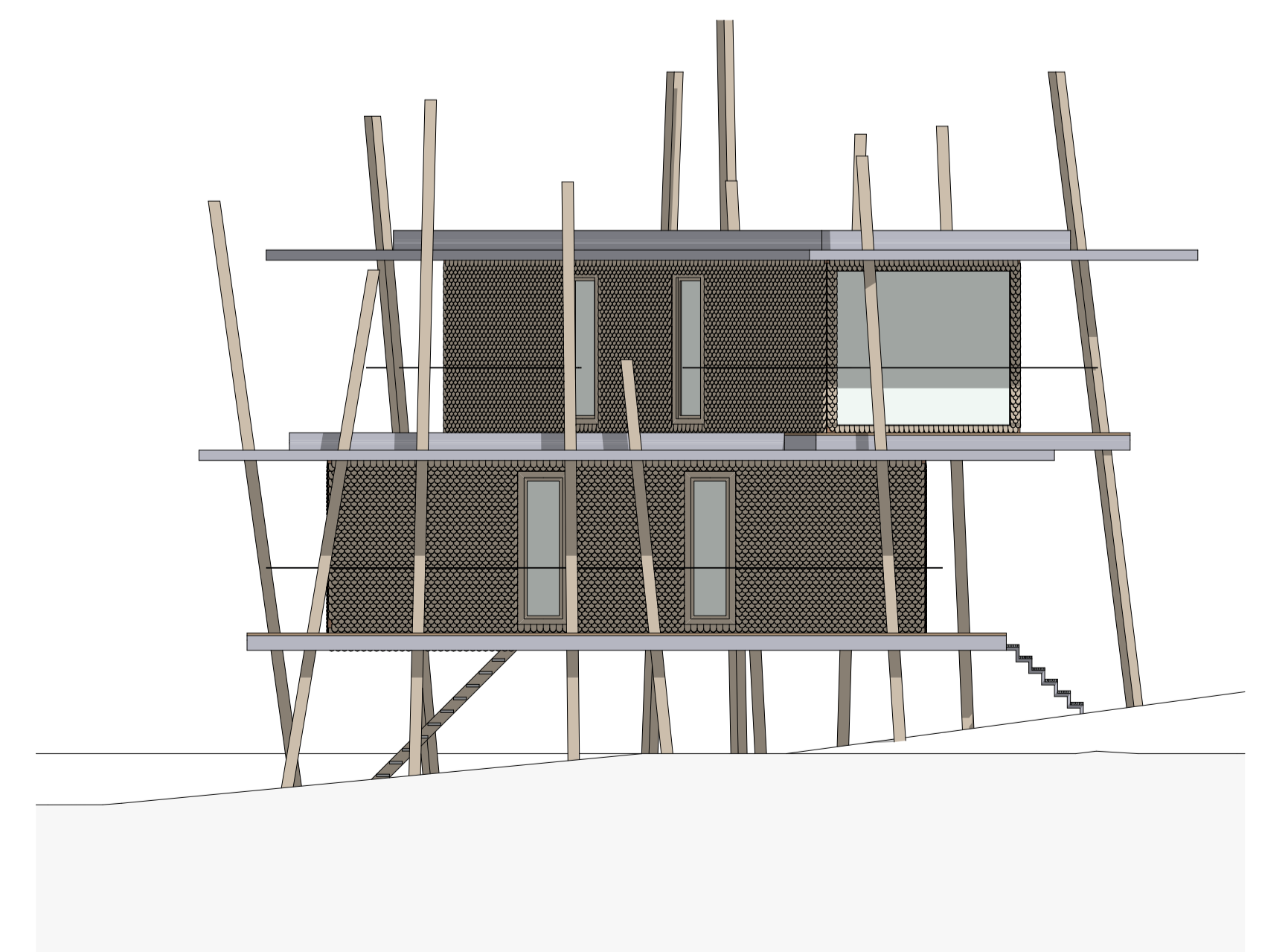
ANSICHT SÜD
